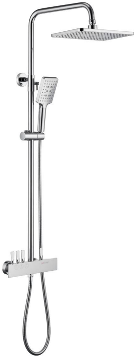
6099-3C 3-Functions shower set Chrome 三功能淋浴花洒 / 铬色
